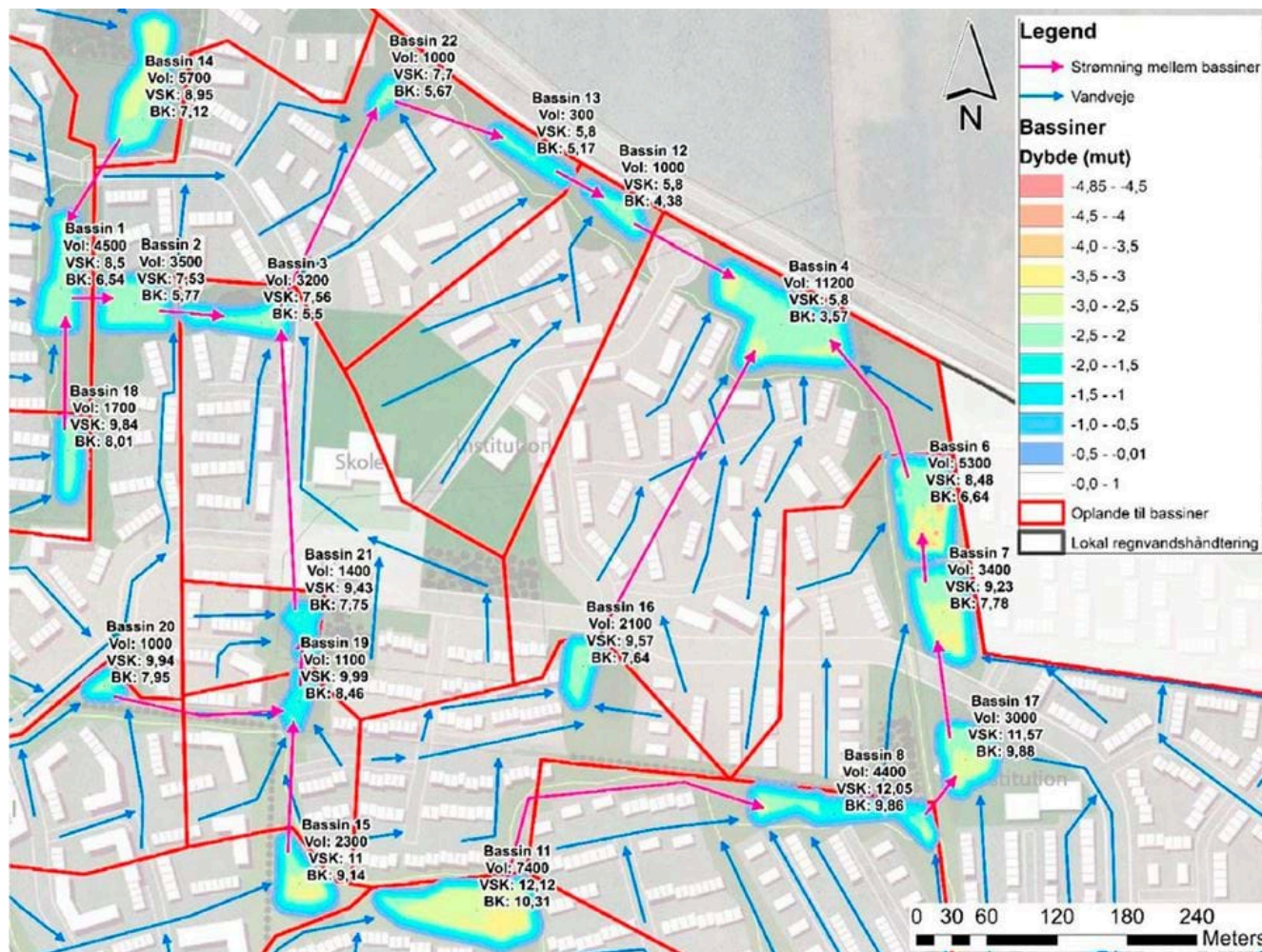
Figur 77: Oversigt over bassiner. Figuren viser placering af bassiner i oplandet, udgravningsdybder og strømningsveje mellem bassinerne. Ud for hvert bassin er der angivet volumen i bassin i m 3 (Vol), maksimal vandspejlskote (VSK) og bundkote i bassin (BK). Fra regnvandshåndteringsplan juni 2024.
